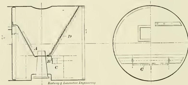
L. S. & M. S. FRONT END.
